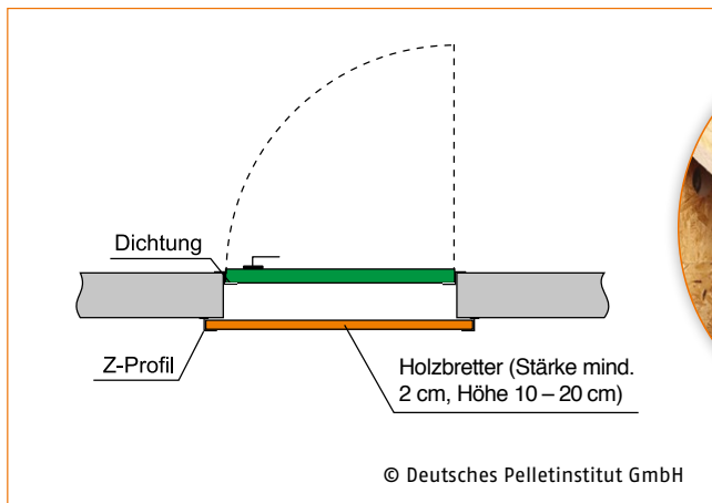
Abb. 20: Druckentlastung der Zugangstür/-luke bzw. Einstiegsöffnung (Draufsicht)
